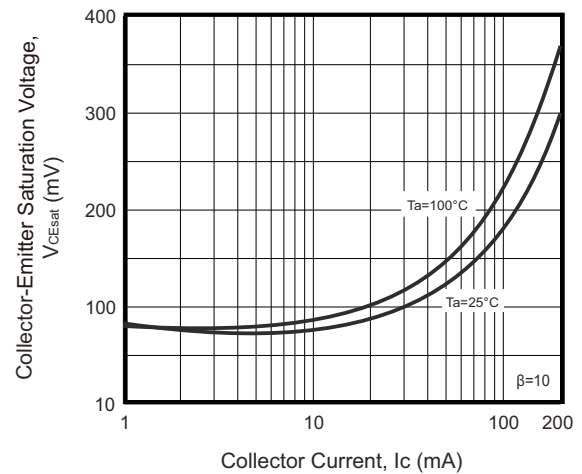
Fig.4 - V_{CEsat} - I_C
