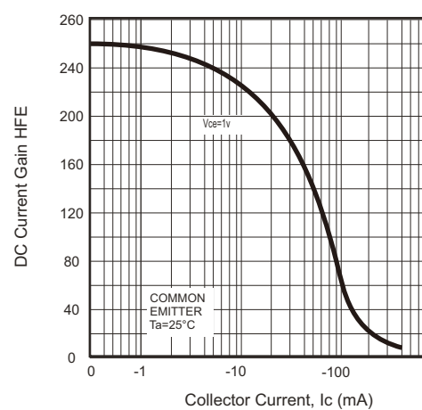
Fig.4 - h_{FE} - I_c
