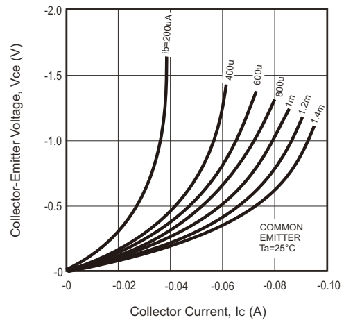
Fig.2 - V_{ce} - I_c
