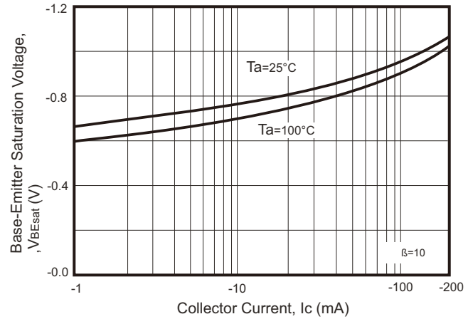
Fig. 4 - V_{BEsat} - I_c
