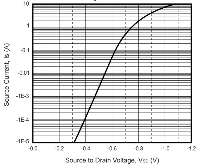
Fig.5 - I_S - V_{SD}
