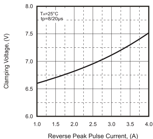
Fig.3 - V_C — I_{PP}
