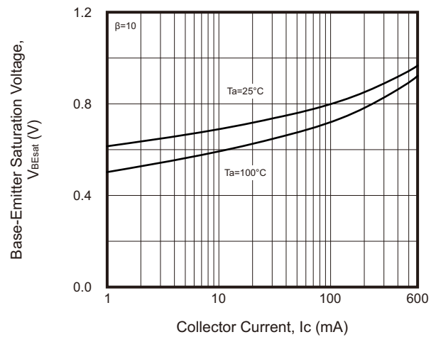
Fig.4 - V_{BEsat} — I_c
