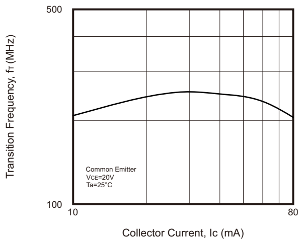
Fig.7 - f_T — I_c
