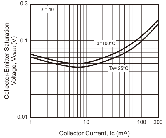
Fig.4 - V_{CEsat} — I_c
