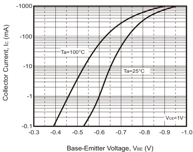
Fig.5 - I_c - V_{BE}
