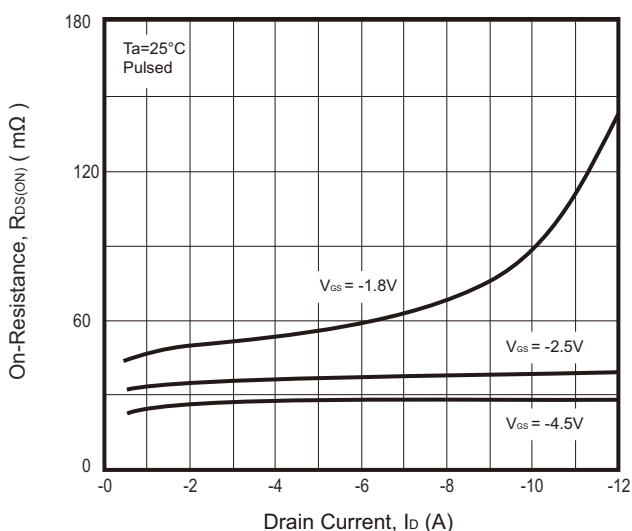
Fig.3 - R_{DS(ON)} - I_D
