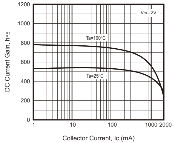
Fig.2 - h_{FE} - I_c
