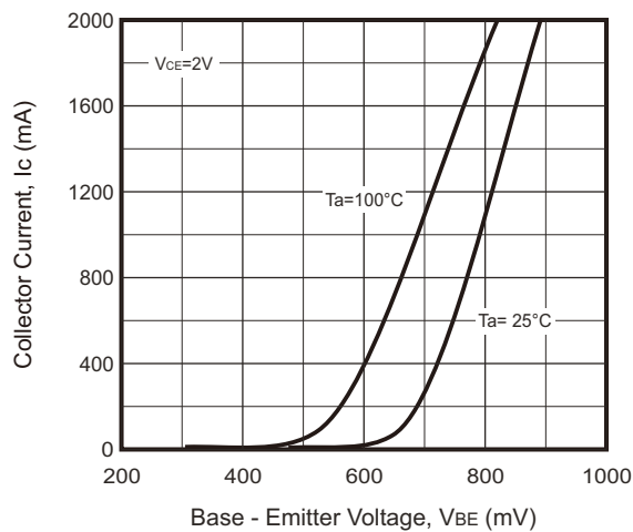
Fig.7 - V_{BE} - I_c
