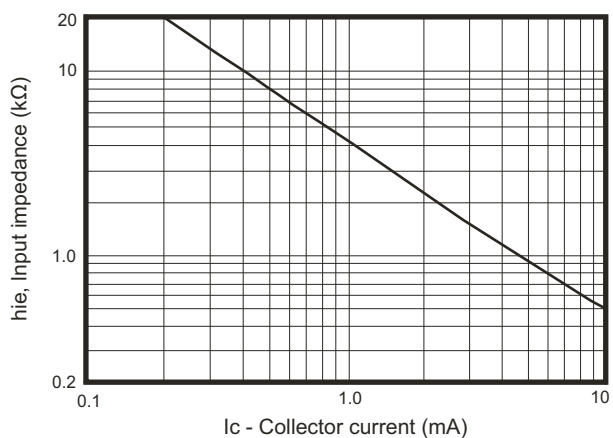
Fig. 9- Input impedance
