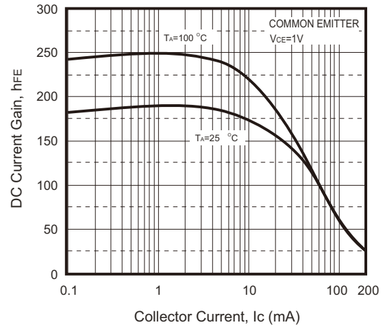
Fig.2 - h_{FE} - I_c
