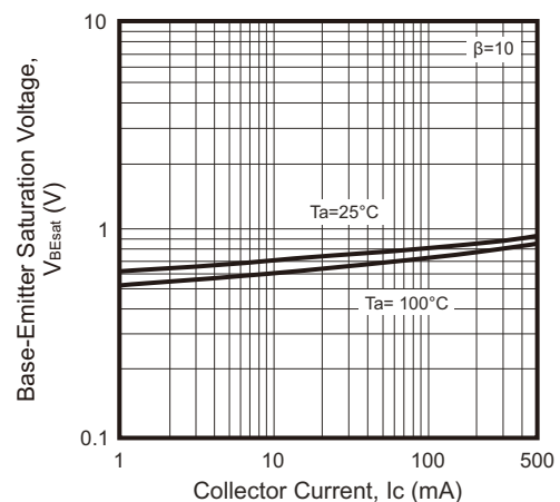
Fig.4 - V_{BEsat} - I_C
