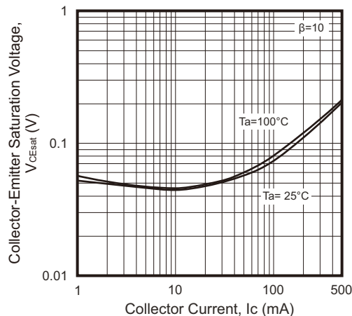
Fig.3 - V_{CEsat} - I_C
