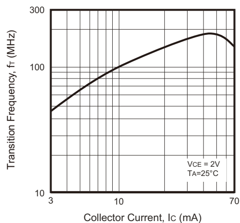
Fig.7 - f_T - I_C
