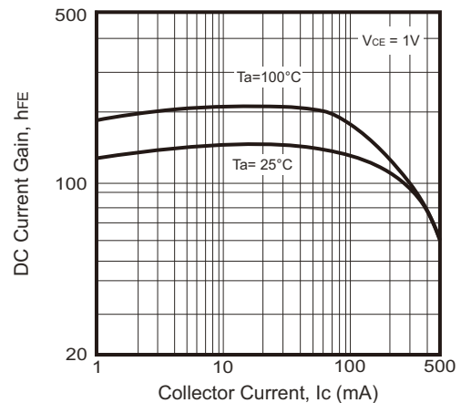
Fig.2 - h_{FE} - I_C
