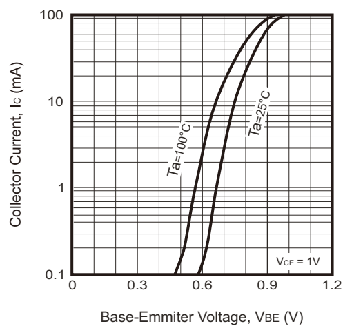
Fig.5 - V_{BE} - I_C
