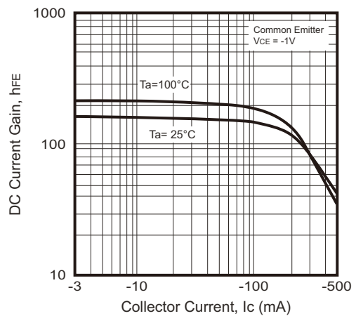
Fig.2 - h_{FE} - I_C
