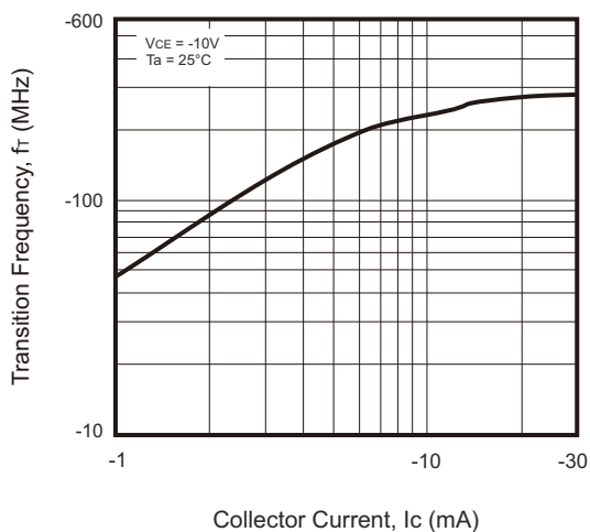
Fig.7 - f_T - I_c
