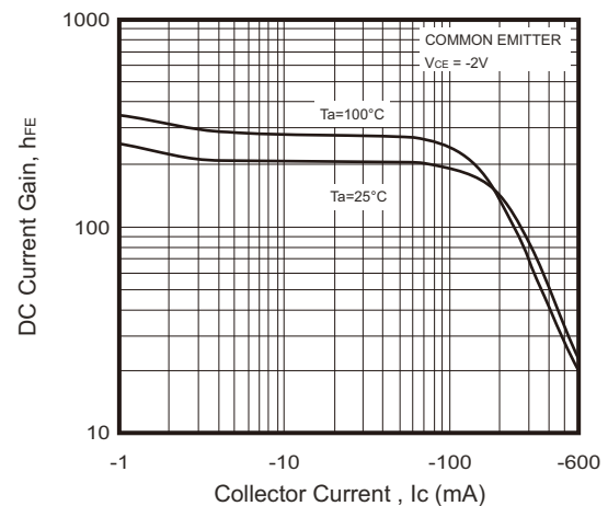
Fig.2 - h_{FE} - I_C
