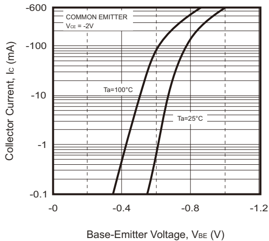
Fig.5 - I_c - V_{BE}
