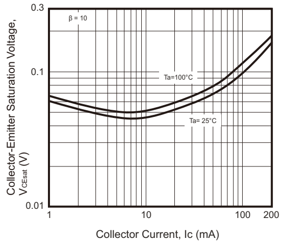
Fig.4 - V_{CEsat} — I_c
