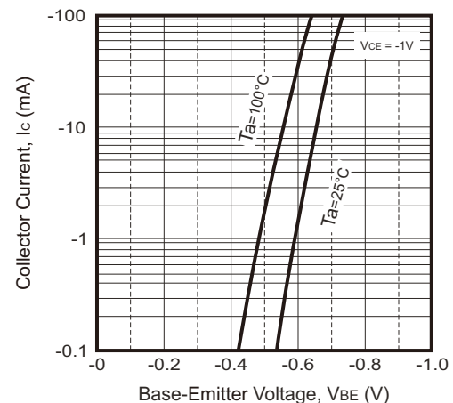
Fig.4 - V_{BE} - I_C
