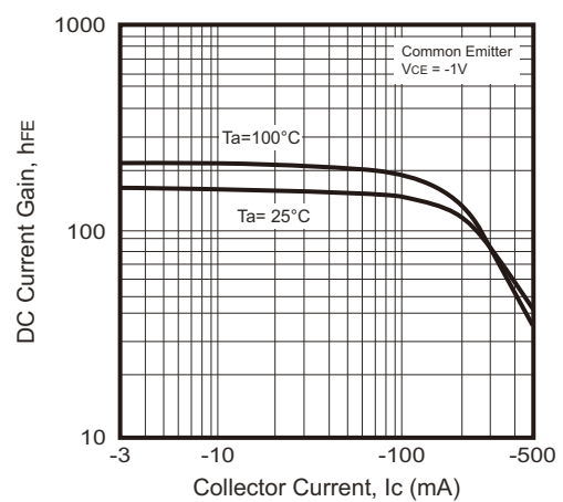
Fig.2 - h_{FE} - I_C
