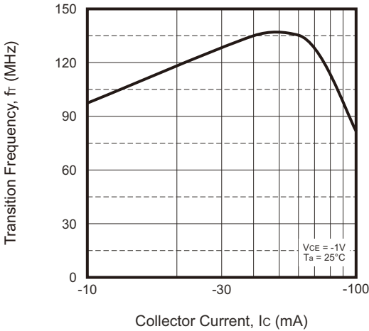
Fig.6 - f_T — I_C
